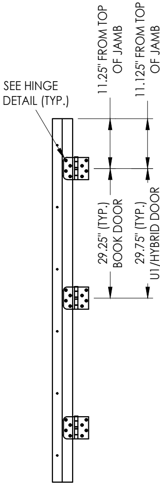
HINGE JAMB
